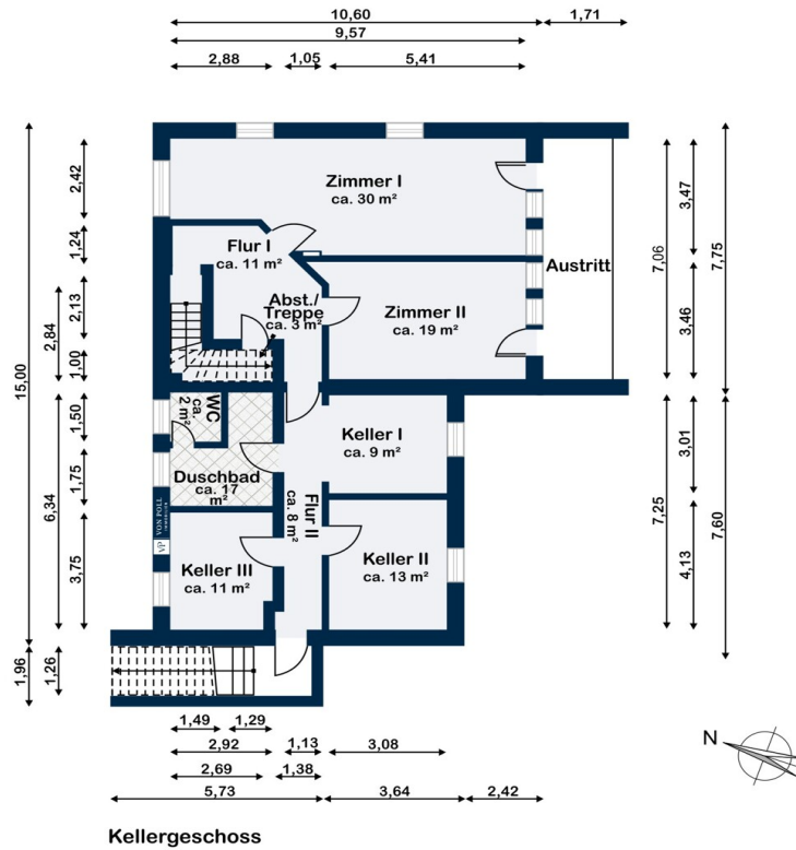
Kellergeschoss
