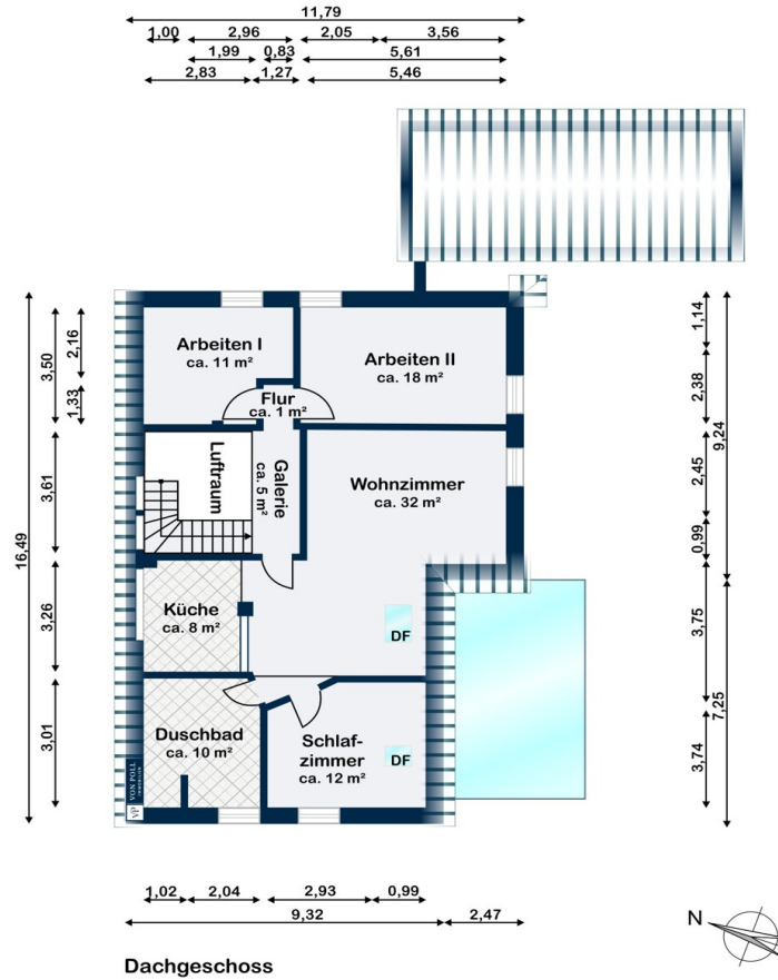
Dachgeschoss
