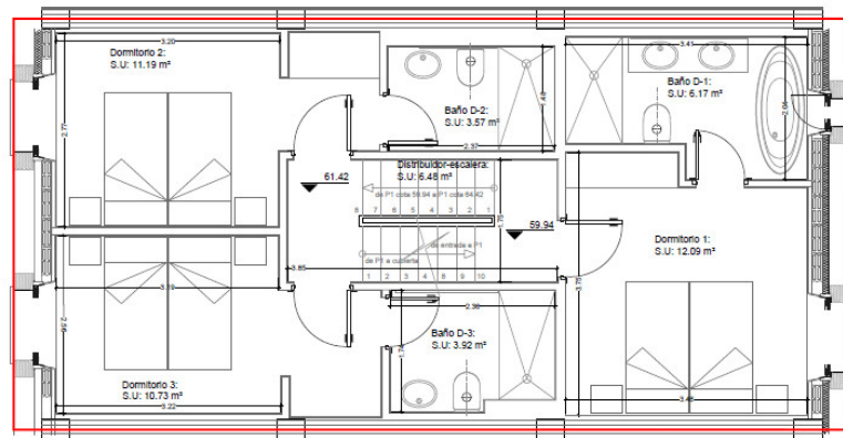
PLANTA PISO
