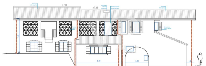
PROSPETTO RETRO
