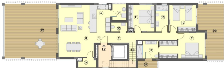
PLANTA SEGUNDA
