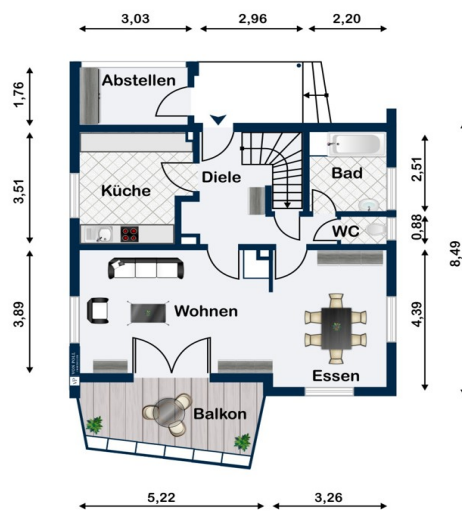
Erdgeschoss
