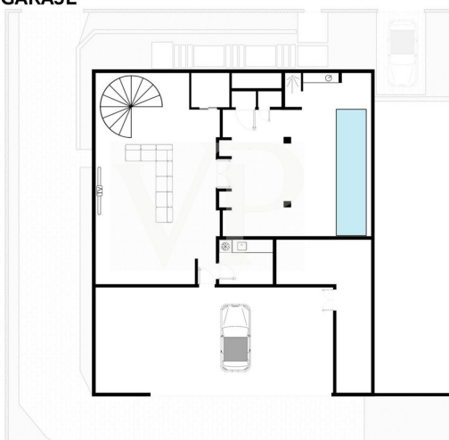
PLANTA -1 / GARAJE
