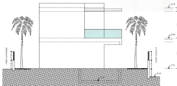
alzado a paseo Alfaneque
