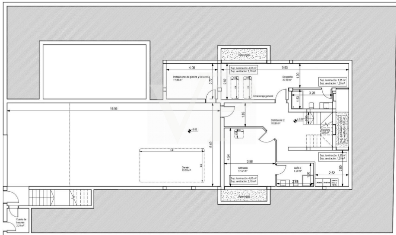
PLANTA SÓTANO
