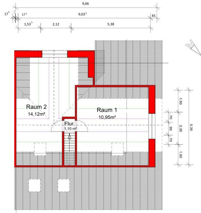
Grundriss Dachgeschoss
