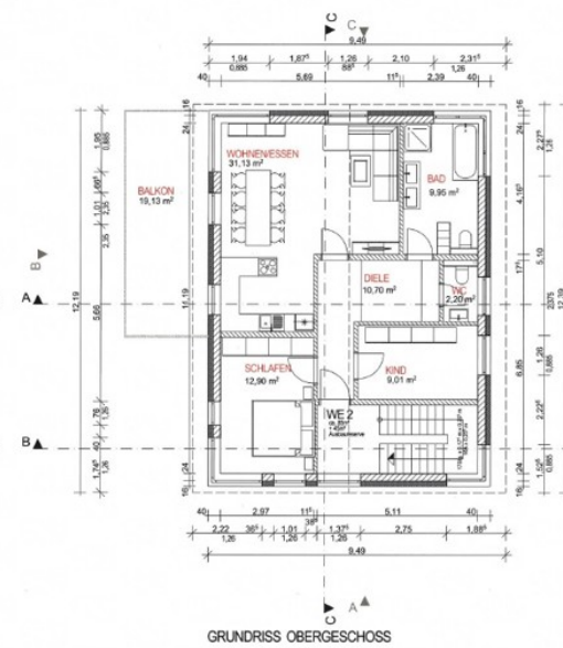
GRUNDRISS OBERGESCHOSS
