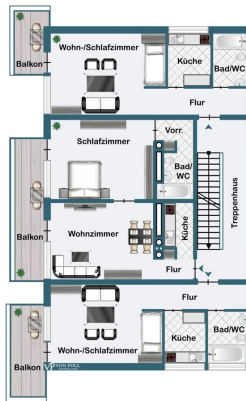
2. Obergeschoss
