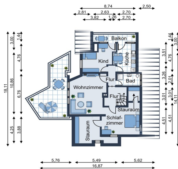
Dachgeschoss
