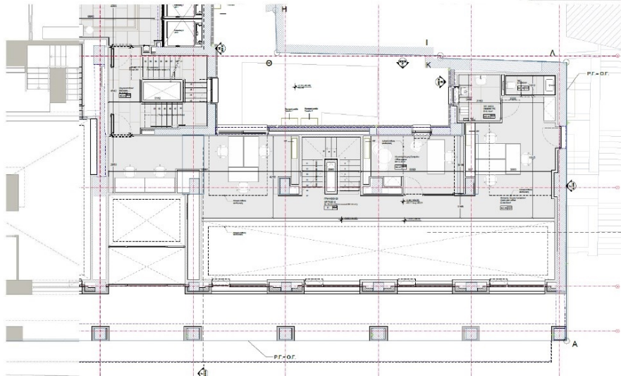
ΚΑΤΩΦΗ ΙΣΟΓΕΙΟΥ ΧΩΡΟΥ ΓΡΑΦΕΙΟΥ 2 / GROUND FLOOR PLAN OF OFFICE SPACE 2
