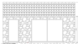
FACHADA POSTERIOR COTA TERRENO NATURAL
