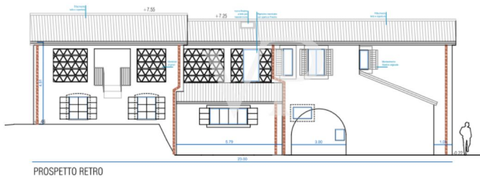
PROSPETTO RETRO
