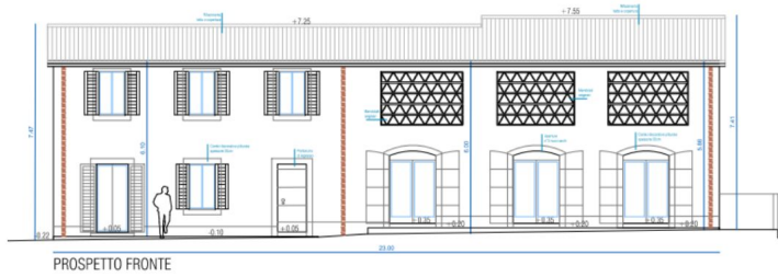
PROSPETTO FRONTE
