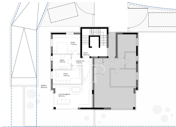
EDIFICIO C, lotto C.2 PIANTA PIANO TERRA - App 01 SCALA 1:100
