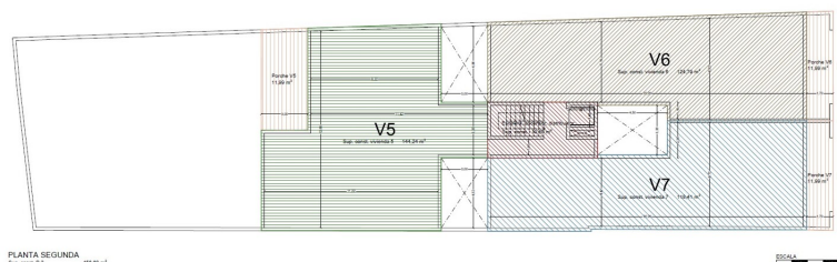
PLANTA SEGUNDA Superficie cubierta: 445,12 m²
