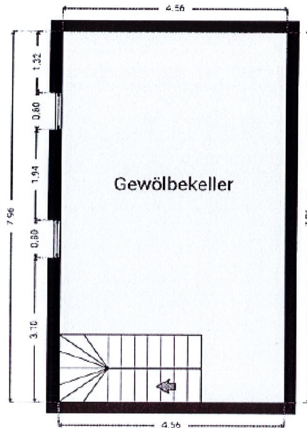
Untergeschoss - Gewölbekeller
