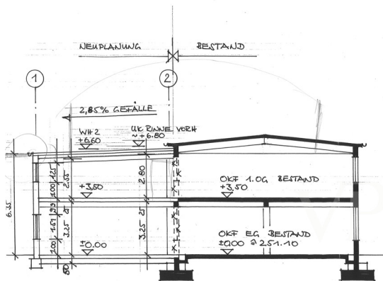
SCHNITT A-A
