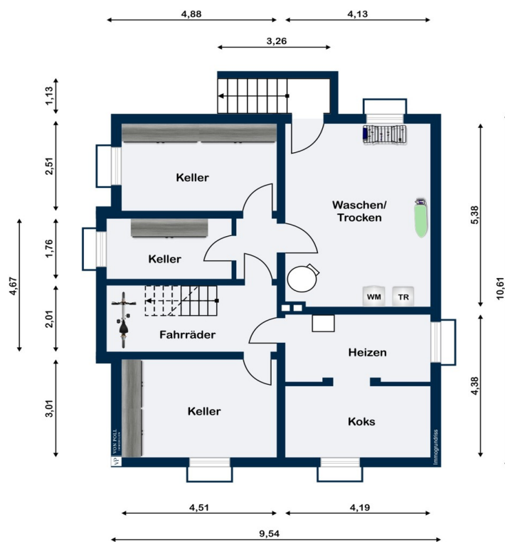
Kellergeschoss
