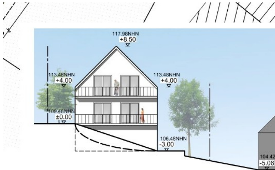
Ansicht Süd/Ost
