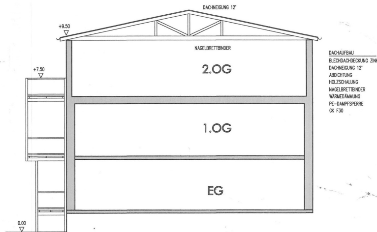
Querschnitt
