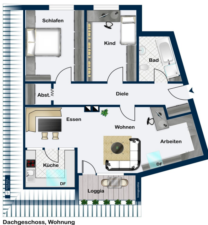
Dachgeschoss, Wohnung
