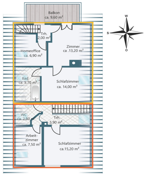
Obergeschoss
