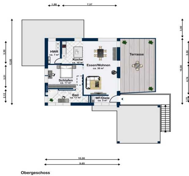
Obergeschoss
