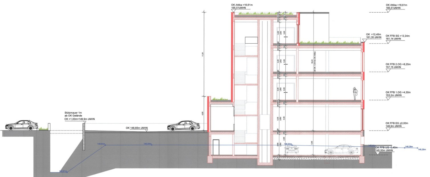
Schnitt C-C
