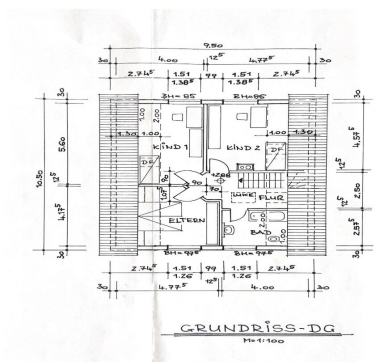
Grundriss Dachgeschoss
