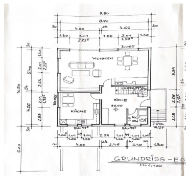
Grundriss Erdgeschoss
