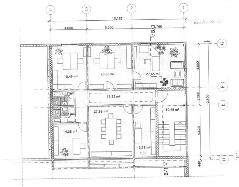
Grundriß Obergeschoß
