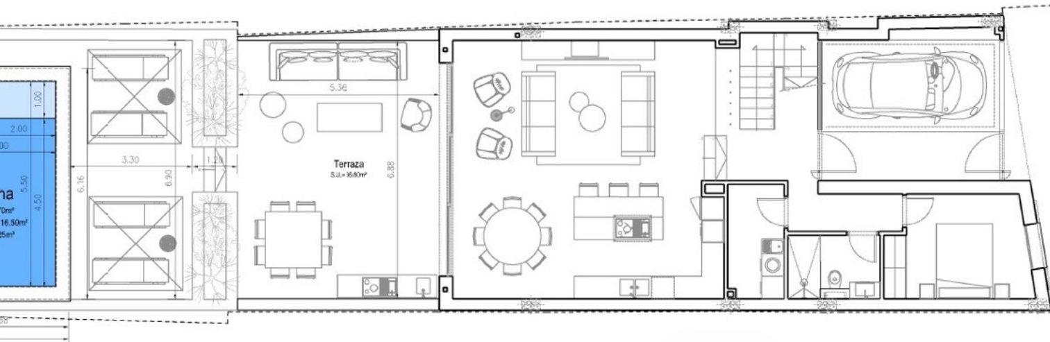
PLANTA BAJA y PISCINA
