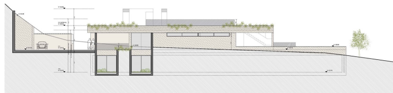
ALZADO 05 - FACIADA SURSE # 1:100-043
