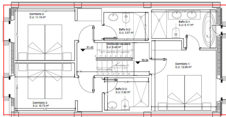
PLANTA PISO
