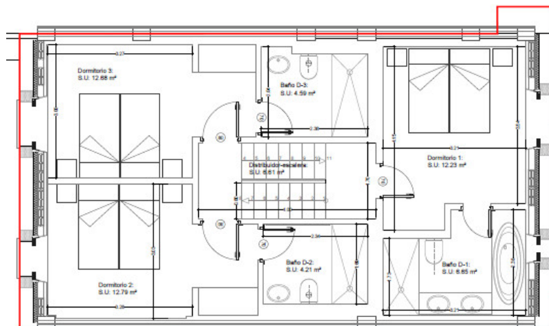
PLANTA PISO
