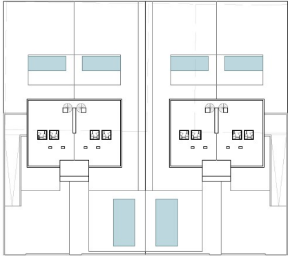
EMPLAZAMIENTO Escala 1:200
