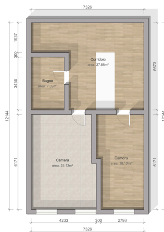
1744_p3 Superficie netta: 79.32m 2
