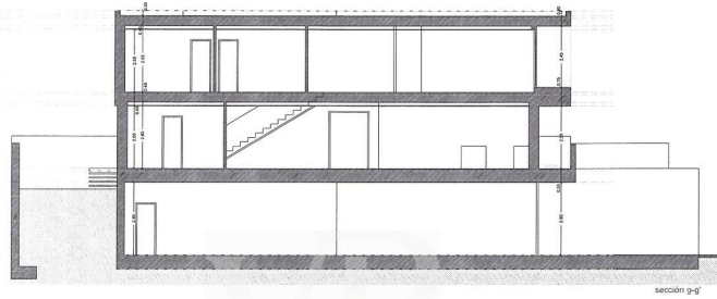
sección g-g'
