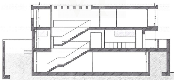
sección h-h'
