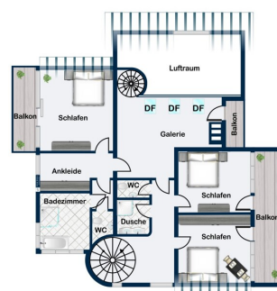
Dachgeschoss
