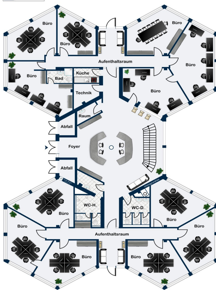
Erdgeschoss
