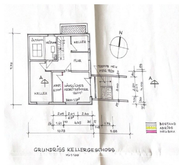
Grundriss Kellergeschoss
