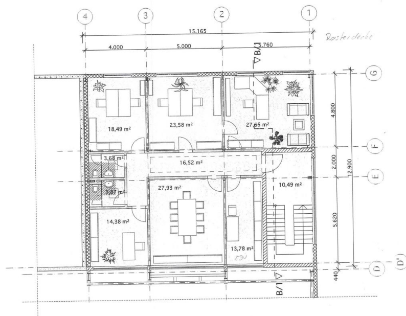
Grundriß Obergeschoß
