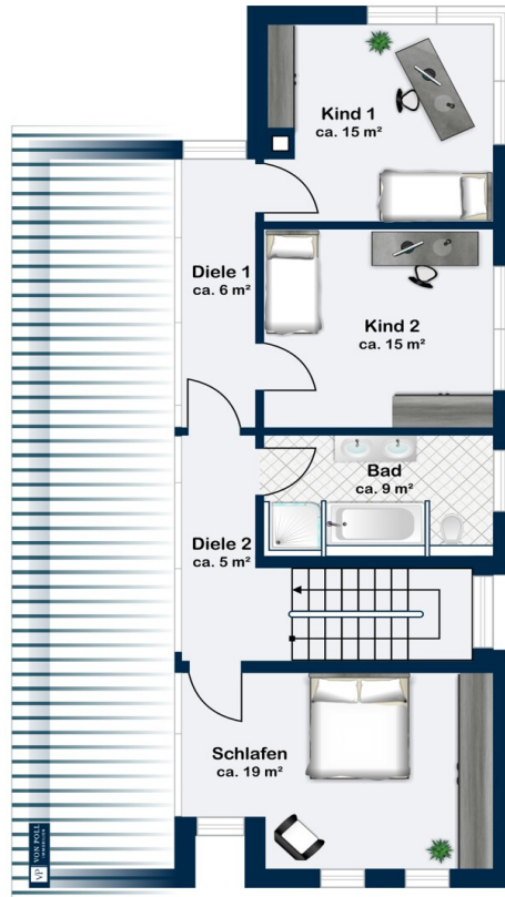
Dachgeschoss
