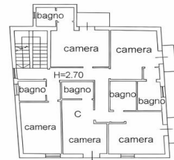
PIANO SECONDO
