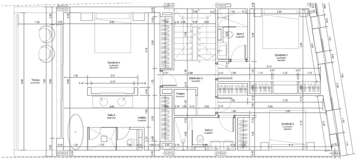
PLANTA PISO
