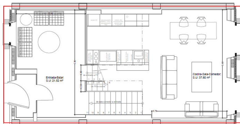
PLANTA BAJA
