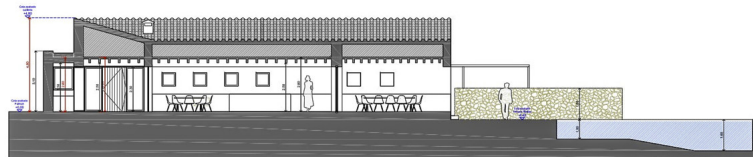
SECCION 1 E: 1/50
