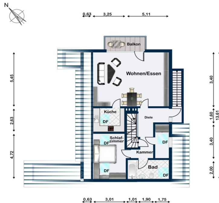
Dachgeschoss
