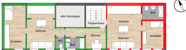
1. Obergeschoss
