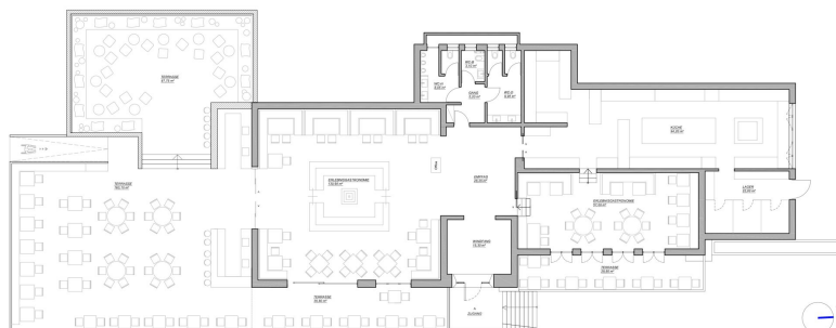
GRUNDRISS ERDGESCHOSS
