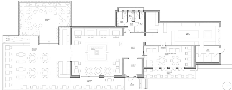
GRUNDRISS ERDGESCHOSS
