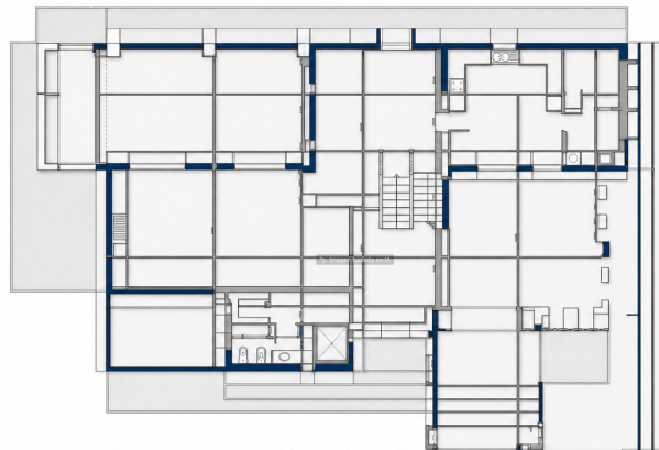
PLANTA ACCESO: cotas
