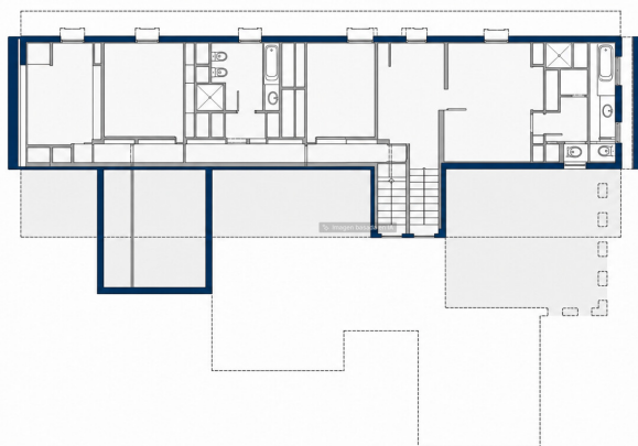
PLANTA DORMITORIOS: cotas
