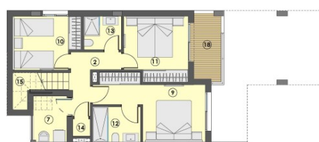
PLANTA SEGUNDA
